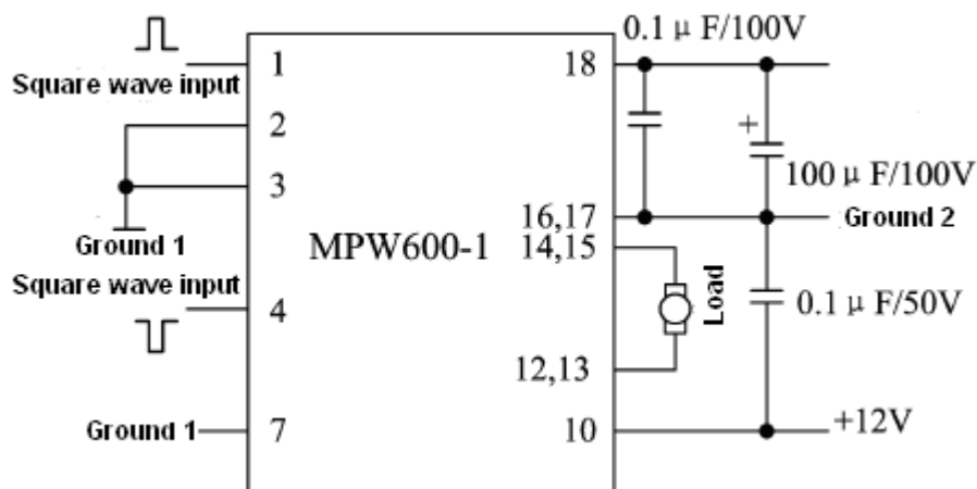
图 4 典型连接图
